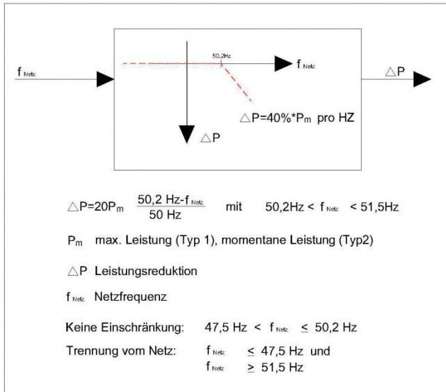
Abbildung 5: Frequenzverhalten von EEA
