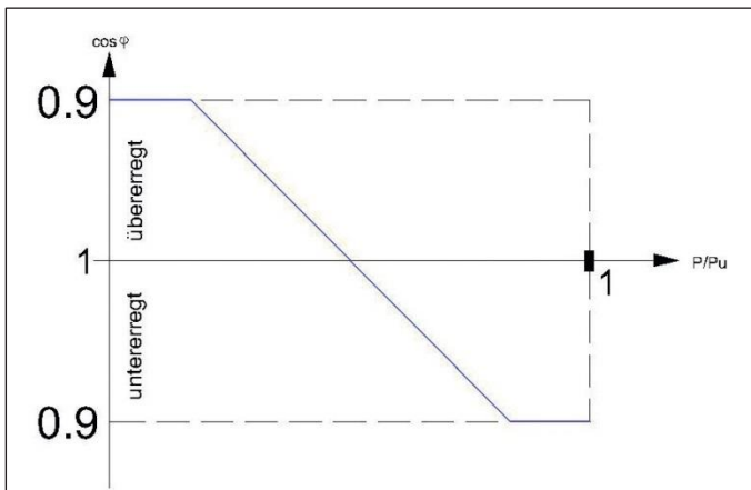
Abb 1: mögliche Blindleistungskennlinie einer EEA
