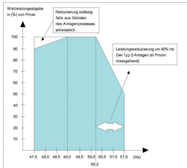
Abbildung 4: Wirkleistungsabgaben in Abhängigkeit der Netzfrequenz
